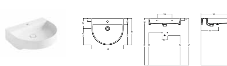
Lavabo 60x51x12H cm - Washbasin - Lavabo
