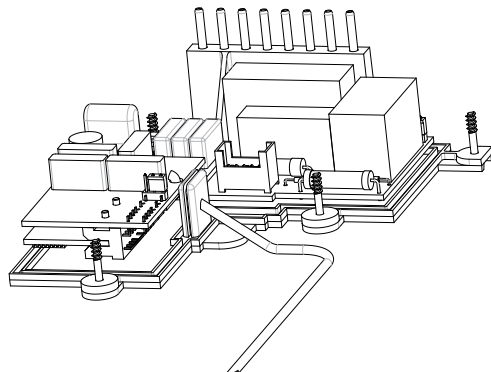
Fig.8-A LIMODOR F/M
