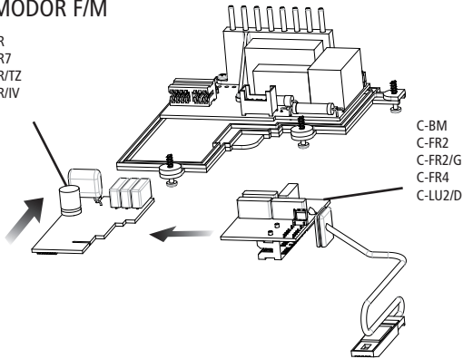
Fig.8-A LIMODOR F/M
